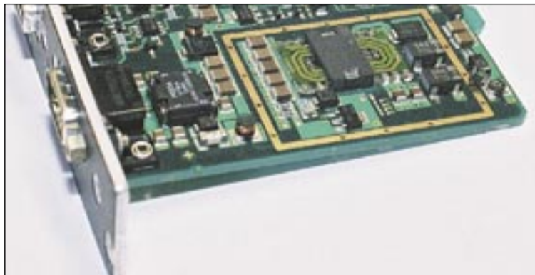
Här ser vi en omvandlare med plan transformator inlagd i kundens konstruktion.
