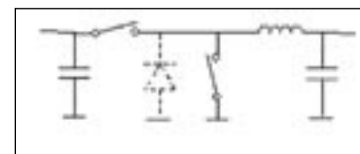
Fig 2. Vid synkron likriktning lägger man en MOSFET (här visad som switch) parallellt över dioden.
