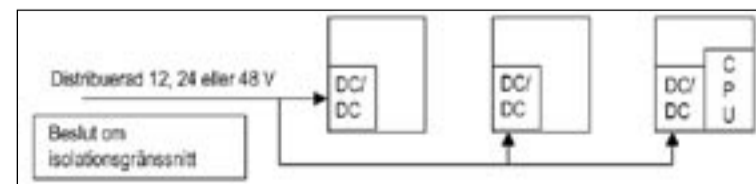
Fig 1. I ett distribuerat kraftsystem måste man först besluta var isolationsgränssnittet skall ligga.
